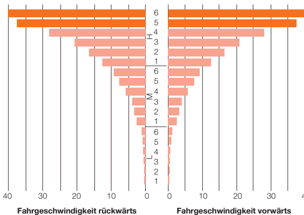
Geschwindigkeitsdiagramm M4003 18V/18R
